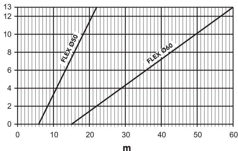
fig. 28 - Grafico per scelta parametro camino
