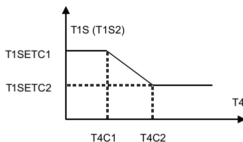
fig. 59 - Curva climatica 9 in modo raffreddamento
